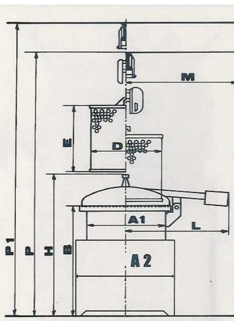
Autoclave Électrique
